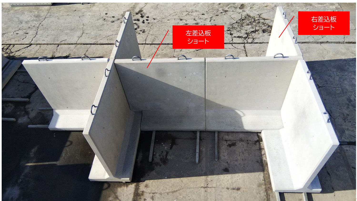
差込（左右）ショートと標準板、左右差込板のレイアウト例
